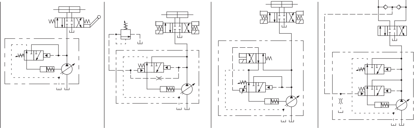
“C**V11B”（*节流口打开） 和“C**V11P”（*节流口堵上）
